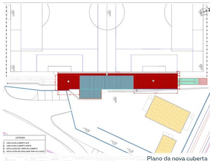
Plano da nova cuberta
